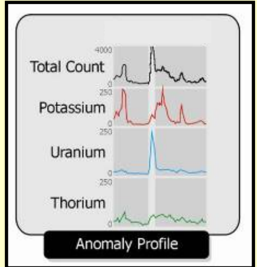
Nungbalgarri Anomaly
